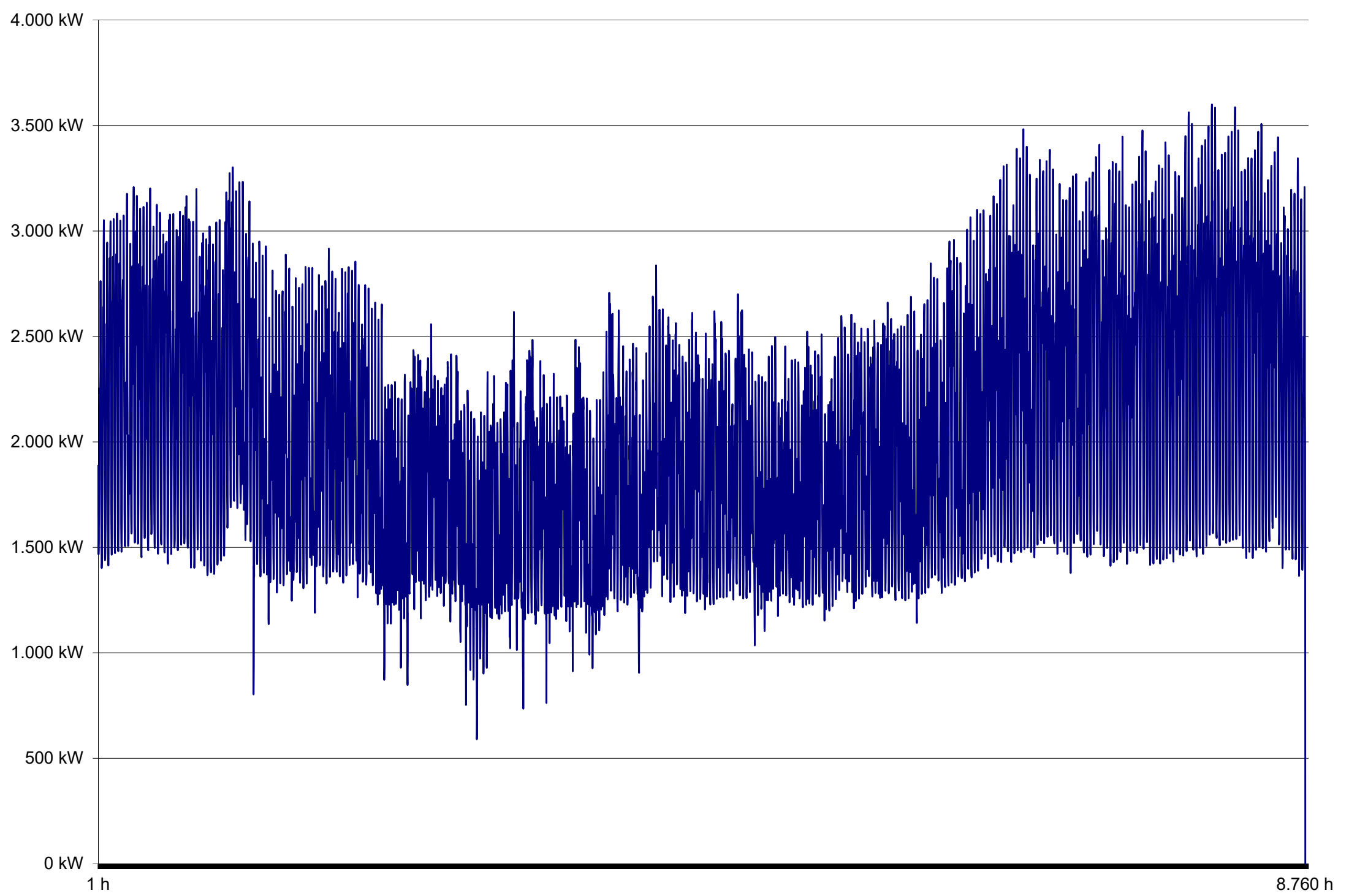
Lastgang Höchstentnahmelast MSP Stadtwerke Deidesheim GmbH 2021
