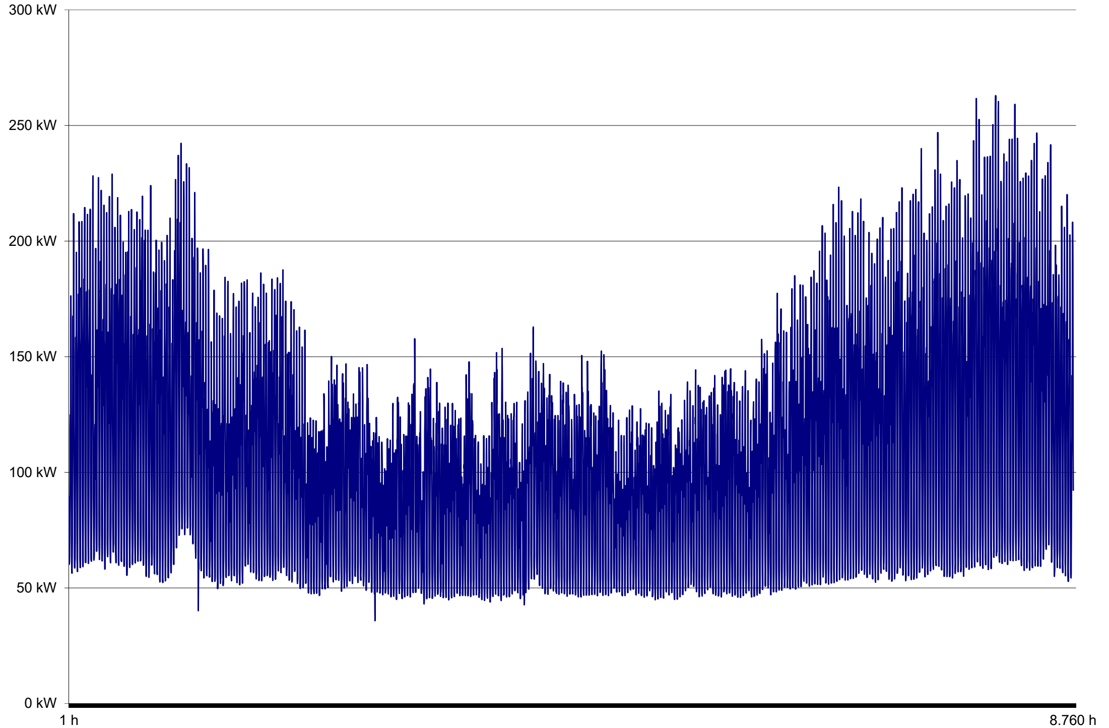
Lastgang Summenlast der Netzverluste Stadtwerke Deidesheim GmbH 2021
