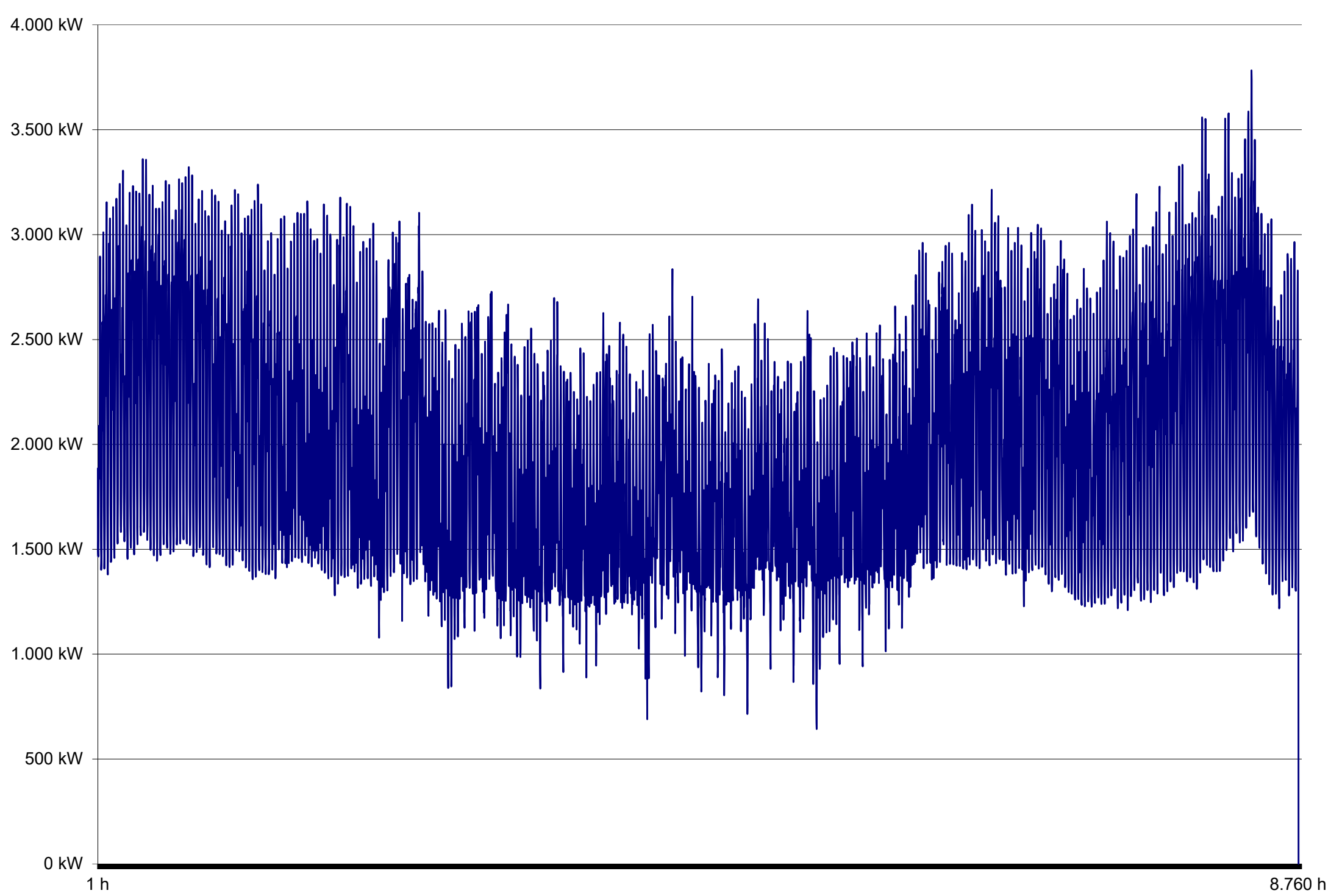
Lastgang Jahreshöchstlast MSP Stadtwerke Deidesheim GmbH 2022
