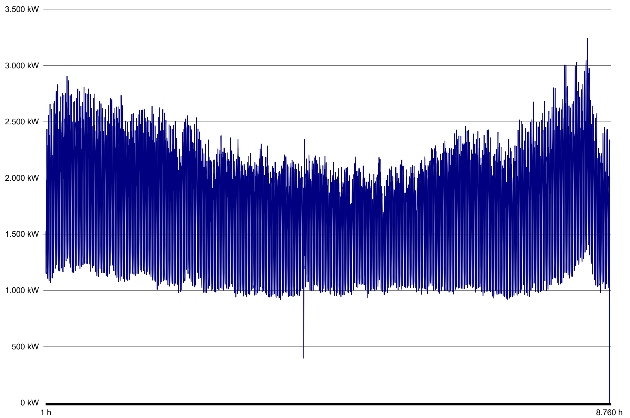
Lastgang Jahreshöchstlast NSP Stadtwerke Deidesheim GmbH 2022
