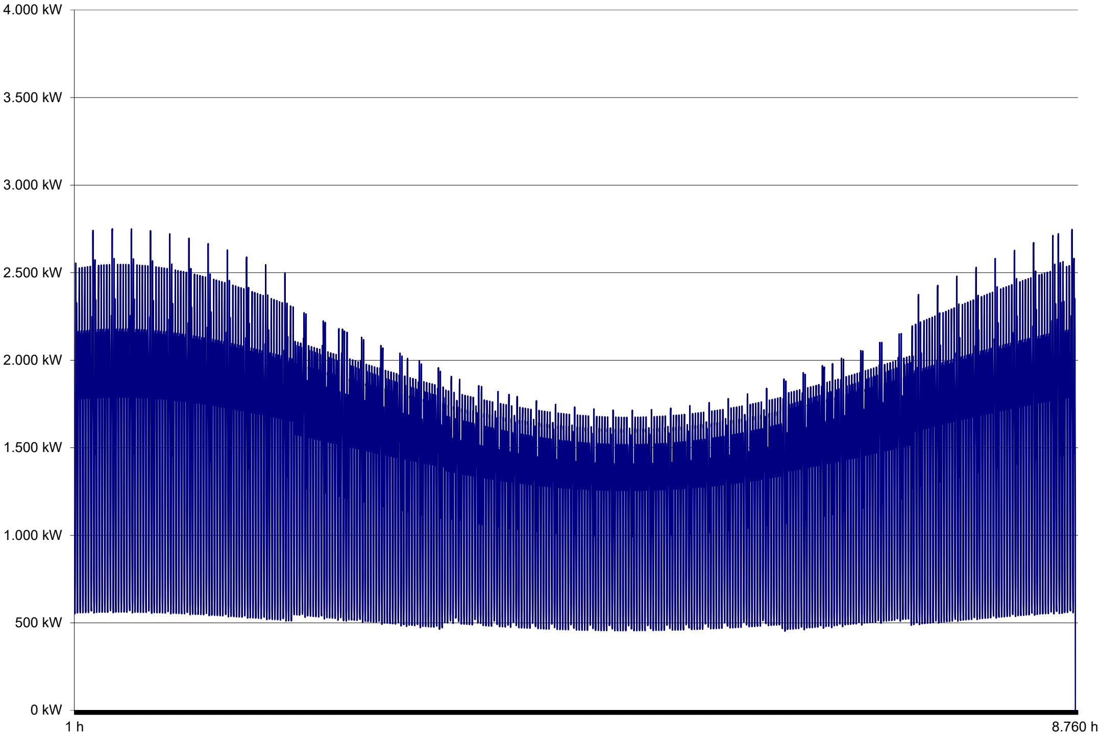
Lastgang der Fahrplanprognosen für Lastprofilkunden Stadtwerke Deidesheim GmbH 2022
